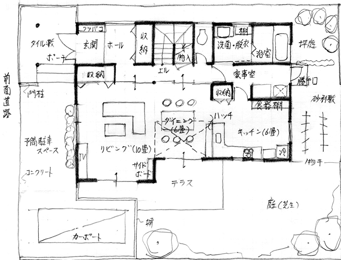
配置図兼1階平面図 1/100
